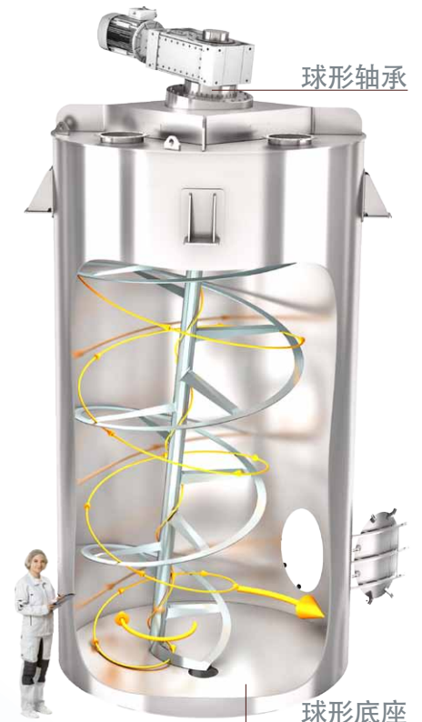
球形轴承 球形底座 两台小型驱动电机就足以精确、轻柔地混合最多 70 立方米的整批物料。
