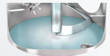
混合设备固定支撑：中心区域的流动较少。因此，旋转频率应超过 4 到 7 转/分钟。
